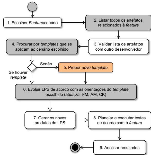
Figura 4. Passos do processo de extração de novas features .
