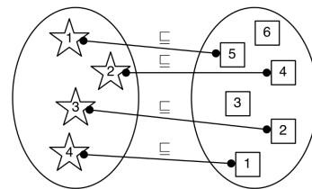
Figura 1. Exemplo ilustrativo do conceito de evolução segura. Elipses representam LPS e seus respectivos produtos.
