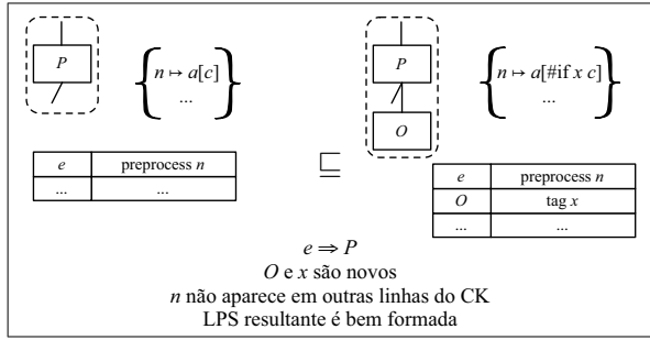
Figura 7. TRANSFORMAR ARTEFATO PRÉ-PROCESSADO EM NOVA FEATURE
