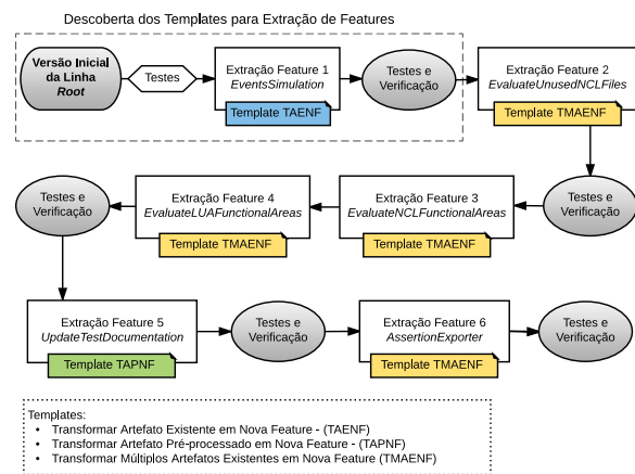
Figura 10. Evolução da nova LPS.
