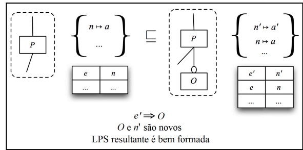
Figura 3. ADICIONAR NOVA FEATURE OPCIONAL [3]
