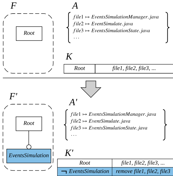
Figura 2. Exemplo: Extrair feature opcional a partir de código existente.
