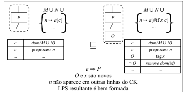
Figura 9. TRANSFORMAR MÚLTIPLOS ARTEFATOS EXISTENTES EM NOVA FEATURE
