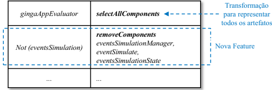
Figura 6. Exemplo de Configuration Knowledge (CK) mais expressivo.
