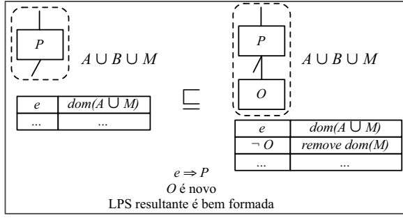
Figura 5. TRANSFORMAR ARTEFATO EXISTENTE EM NOVA FEATURE
