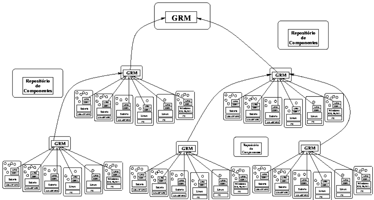
Figura 3: Hierarquia de agrupamentos
