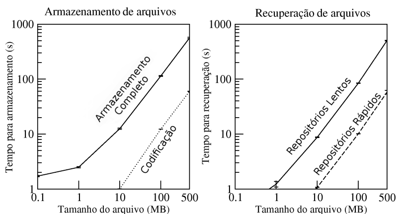
Figure 3. Armazenamento e recuperação de dados armazenados em máquinas remotas.
